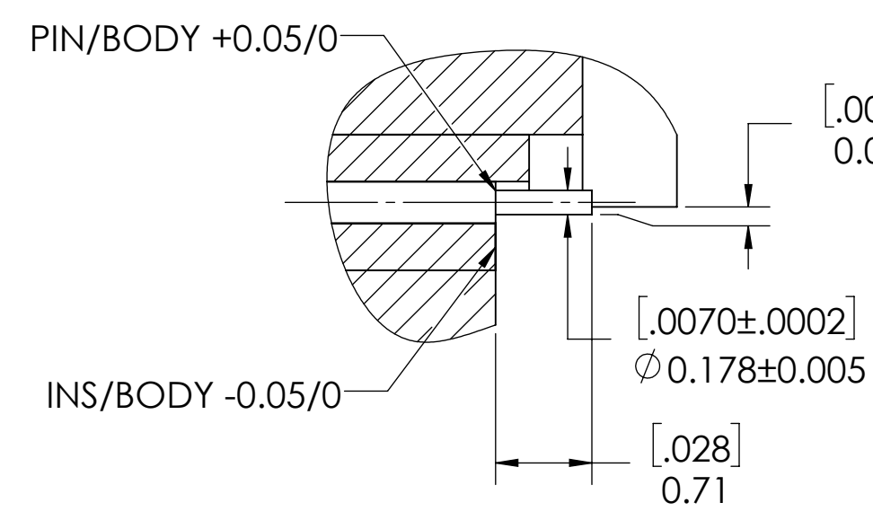
SECTION A-A SCALE 20 : 1
