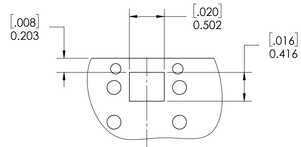
LAYER 3 CUTOUT
