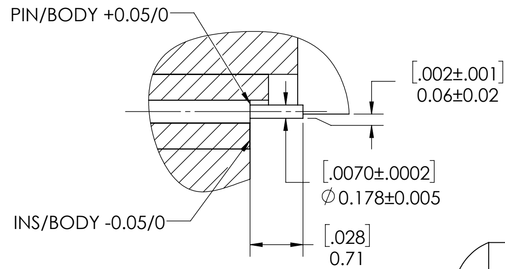
SECTION A-A SCALE 20 : 1
