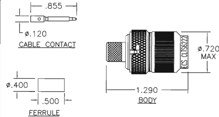
DIMENSIONS \Delta
