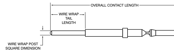
Wire Wrap Contact
